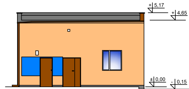
ELEWACJA ZACHODNIA - BUDYNEK E
